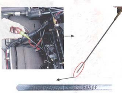
オイルをウエスでふき取り、差し込んでからもう一度 引き抜きオイルの量を確認 ゲージに付着したオイルを指で触って確認
