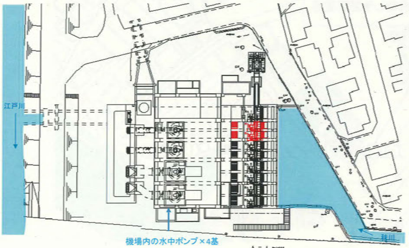
平面図(秣川排水機場(赤印が除塵機2号・3号))
